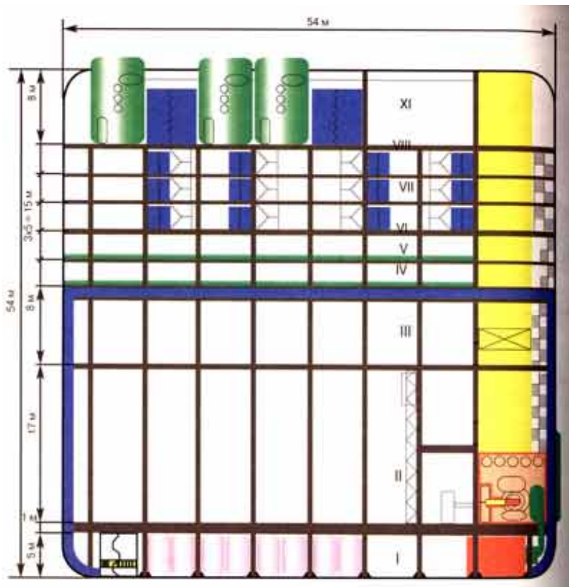
Вертикальное сечение секции корабля "Страж небес"
