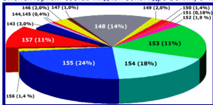
Элементарный состав жидкой зоны ядра Земли, в %
