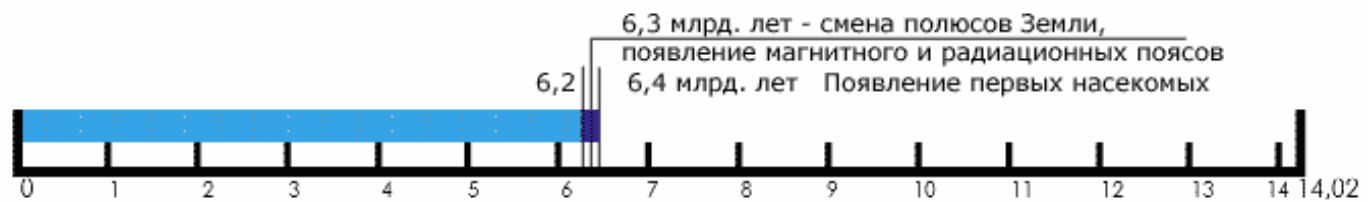
цикл развития Солнечной системы, миллиардов лет
