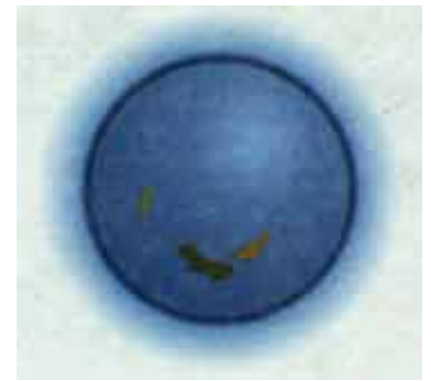
Начало формирования материков
