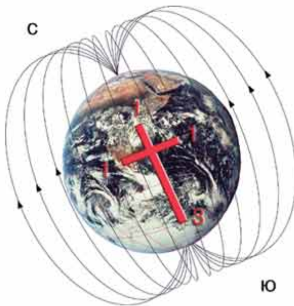
Графическое изображение вектора напряжённости витонного поля Земли
