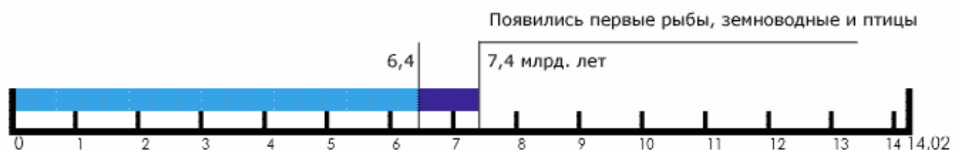
цикл развития Солнечной системы, миллиардов лет
