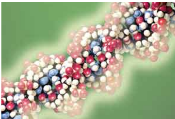
Фрагмент молекулы ДНК с полупрозрачной оболочкой витонной матрицы - живая материя.
