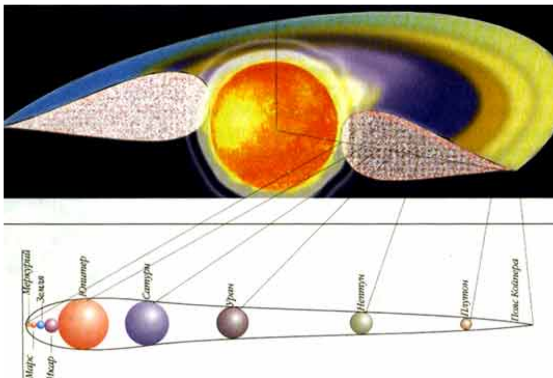
Схема распределения материи в пространстве будущей Солнечной системы
