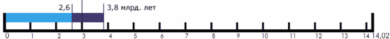
цикл развития Солнечной системы, миллиардов лет
